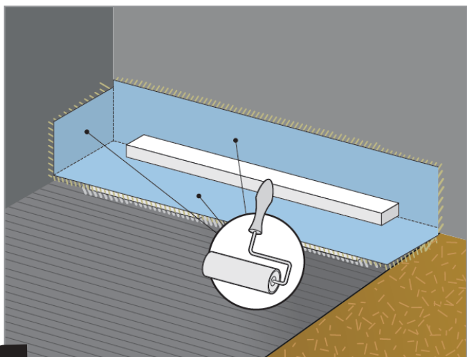
13 Bed the membrane down onto a tile adhesive (EN 12004 C2).
